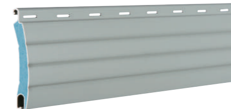
ALUMINIUM DOUBLE PAROI MOUSSE PU Densité - 350kg/m 3
